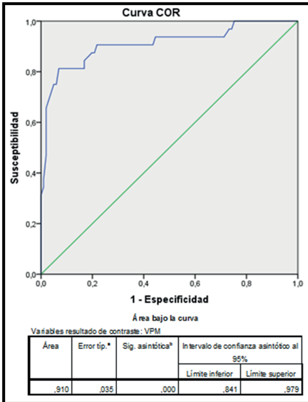
Figura 1. Curva ROC del volumen plaquetario medio para el diagnóstico de infarto agudo de miocardio sin elevación del ST.
